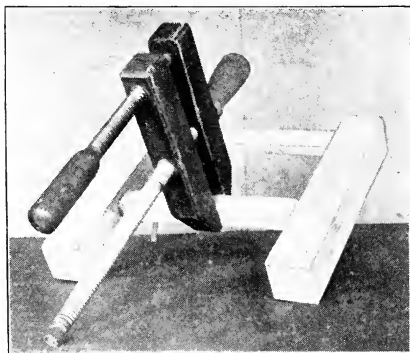
Fig. 223—Turning Rung
